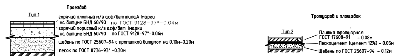
Конструкция дорожной одежды
